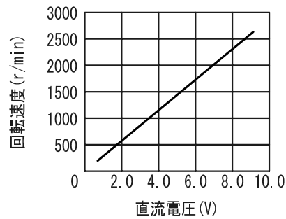
直流電圧・回転速度、参考特性
